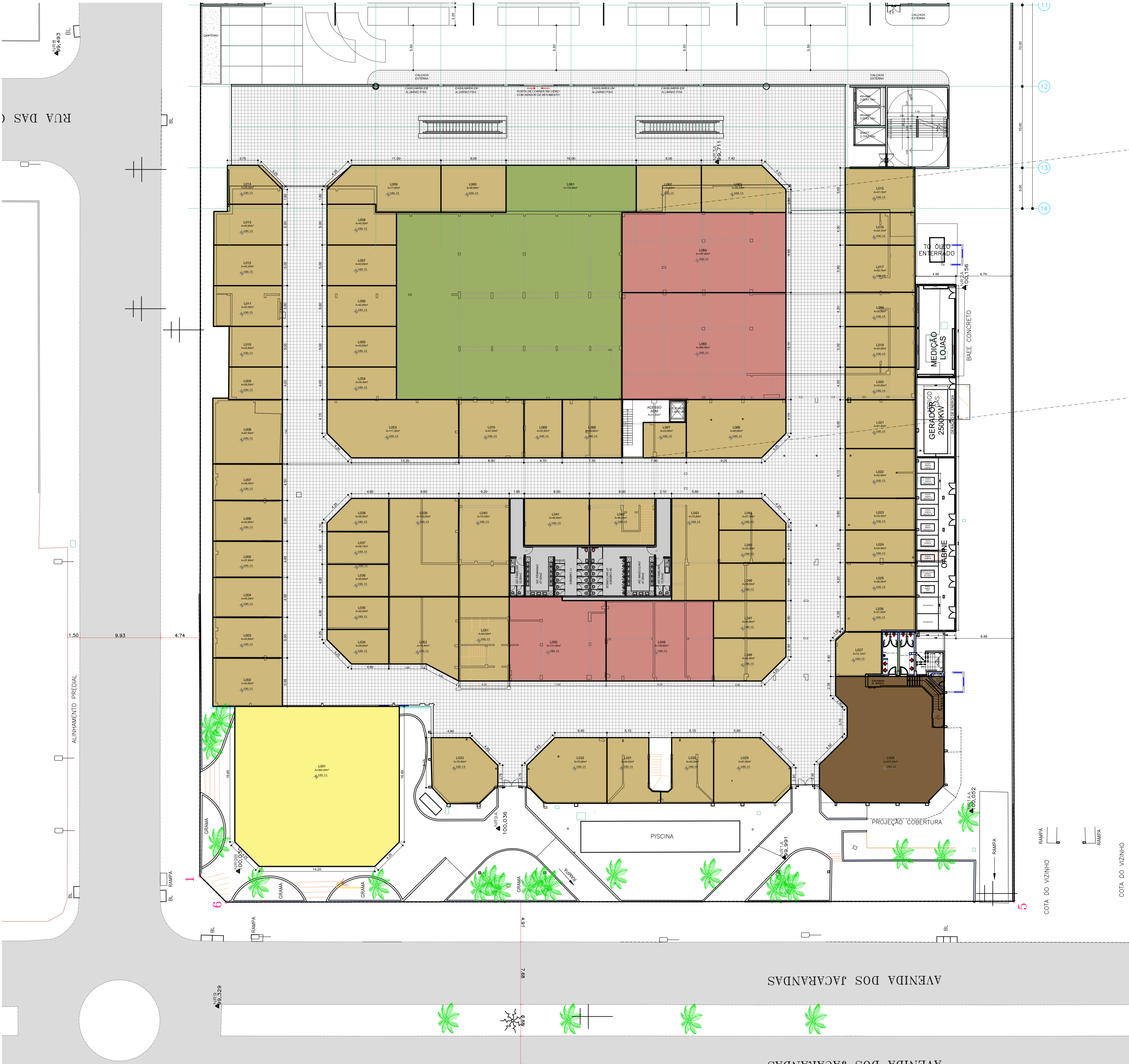
01 PLANTA DO TÉRREO 001 1/250
